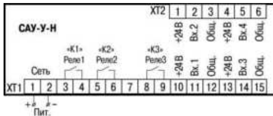
Рисунок 5.1 – Клеммник SAU-Y-N
