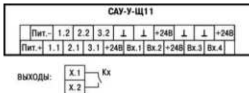
Рисунок 5.2 – Клеммник SAU-Y-Щ11
