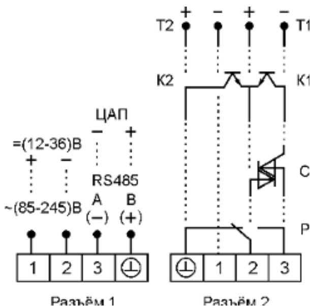
Рис. 4.1 Схема подключения
