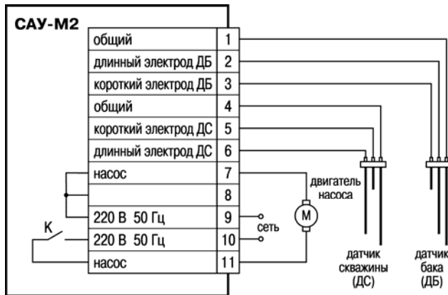
Рисунок Б.1 – Подключение САУ-M2 при использовании для заполнения резервуара с помощью погружного насоса с защитой от «сухого хода»
