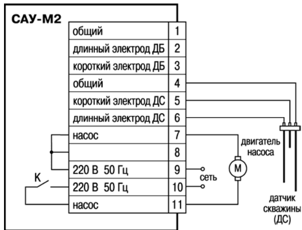
Рисунок Б.2 – Подключение САУ-М2 при использовании для осушения
