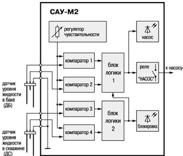
Рисунок 3.1 – структурная схема прибора
